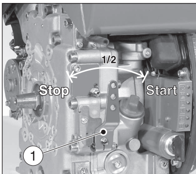
1 Drehzahlverstellhebel
