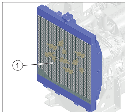
1 Kühlerlamellen
