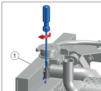
1 Schlauchklemme
